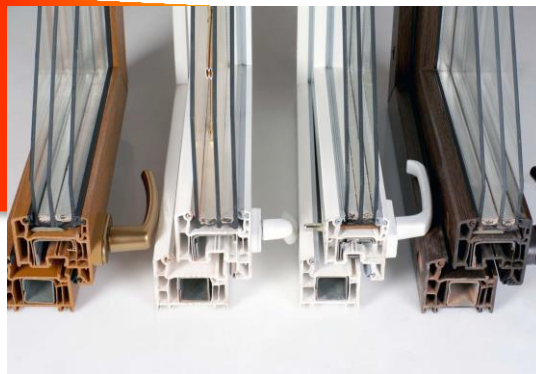
Cadre PVC - Aluminium
